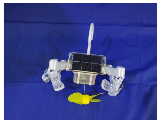
丸善製薬賞 「ソーラー乾燥ハンガー」 広島大学附属中学校 1年生の作品
